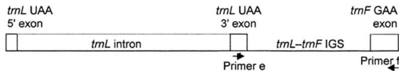
Fig. 1. cpDNA trnL -F region (Pirie et al. 2007).
